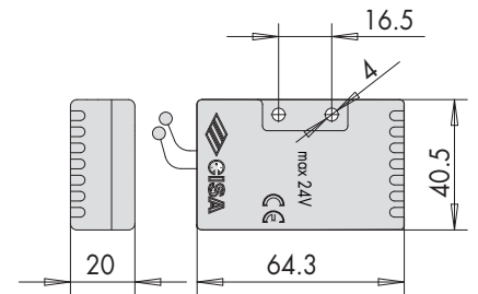
ARTÍCULO 07022.00.0
