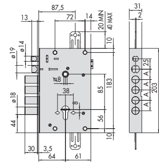
SERIE 15515, 17515, 17665 A = 28
