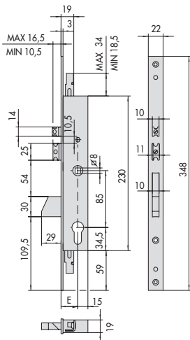
SERIE 16225 E = 25 - 30 - 35
