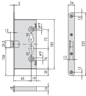
ARTÍCULO 43000.65, 43110.65, 43160.65
