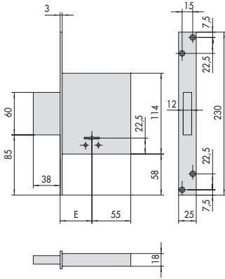
SERIE 57010 E = 52 - 60 - 70
