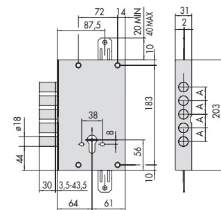
SERIE 57505, 57506, 57655, 56505 A = 28
