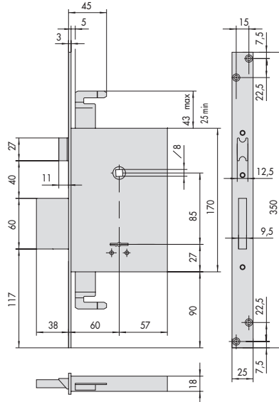
SERIE 57255
