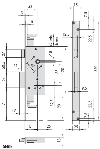
SERIE 57215 E = 45 - 50 - 60
