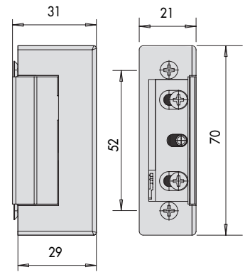
ARTÍCULO 15100, 15101, 15110, 15120, 15121, 15130, 15140, 15150
