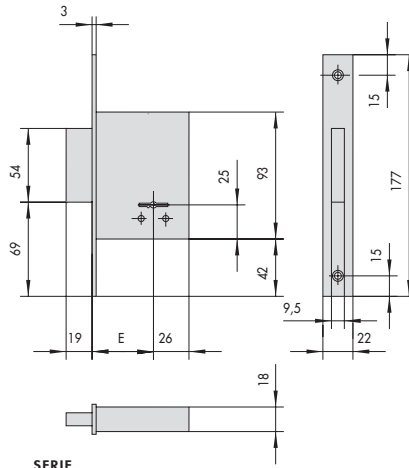
SERIE 57220 E = 40 - 45 - 50 - 60
