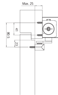
Lado opuesto bisagras (posición invertida)
