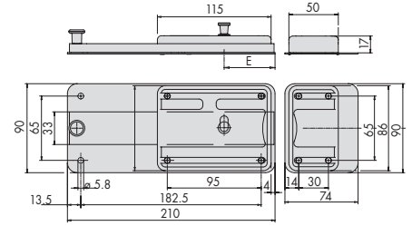
ARTÍCULO 55051, 55054, 55071, 55074 E= 50-60
