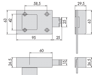
ARTÍCULO 54570.60
