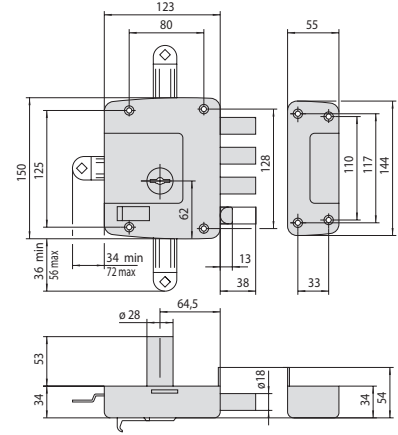
ARTÍCULO 57152.60, 57157.60, 57162.60, 57167.60, 57172.60, 57177.60
