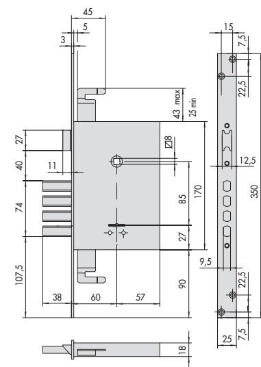
SERIE 57265
