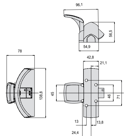
ARTÍCULO 59051, 59061, 59066
