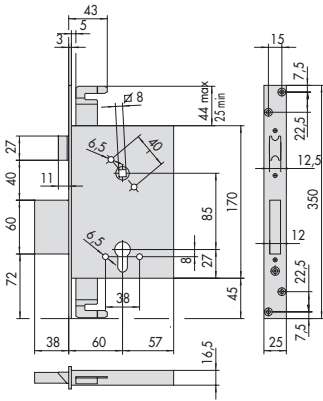
ARTÍCULO 56255.60
