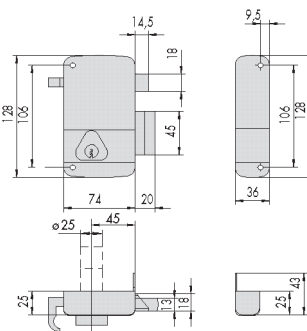
ARTÍCULO 50220.45, 50221.45
